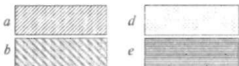
3.10-rasm. Sifatli rang (fon) usuli. Tekislik tuproqlari: a) bo'z qo'ng'ir cho'l; b) cho'l taqir tuproqlari, taqirlar; d) sho'rxoklar; e) qayir (allyuvial).
