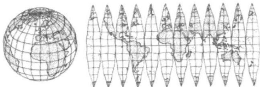
2.3-rasm. Meridianlar bo'yicha zonalarga (tilimlarga) bo'lingan globus yuzasi. Yerning egri yuzasini tekislikda uzilishsiz tasvirlab bo'lmashligini tasdiqlovchi sxema.
