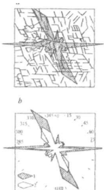
12.7-rasmda keltirilgan roza-diagrammaning nurlari tegishli azimutlar uzunligiga proporsional.
