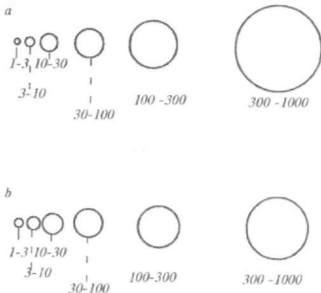
3.20-rasm. Belgilarning pog'onali shkalasi. a — absolyut; b — shartli ko'rsatkichlarda.
