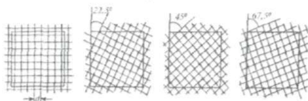
12.12- rasm. Kvadratli paletka yordamida egri chiziqlarning umumiy uzunligini aniqlash.
