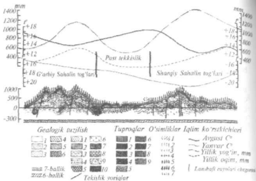
12.6-rasm. Saxalin orolining ko'ndalang kompleks profili.
