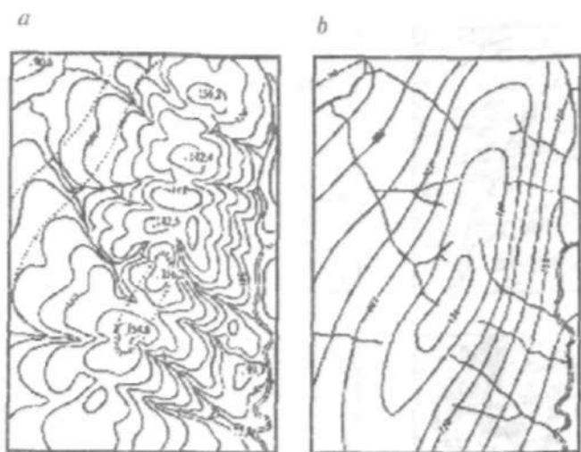
13.5-rasm. Soddalashtirish. Zamonaviy relef kartasini morfo-izogips kartasiga aylantirish: a — zamonaviy relef; b — umumlashgan gorizontallar yordamida relefni tasvirlash.
