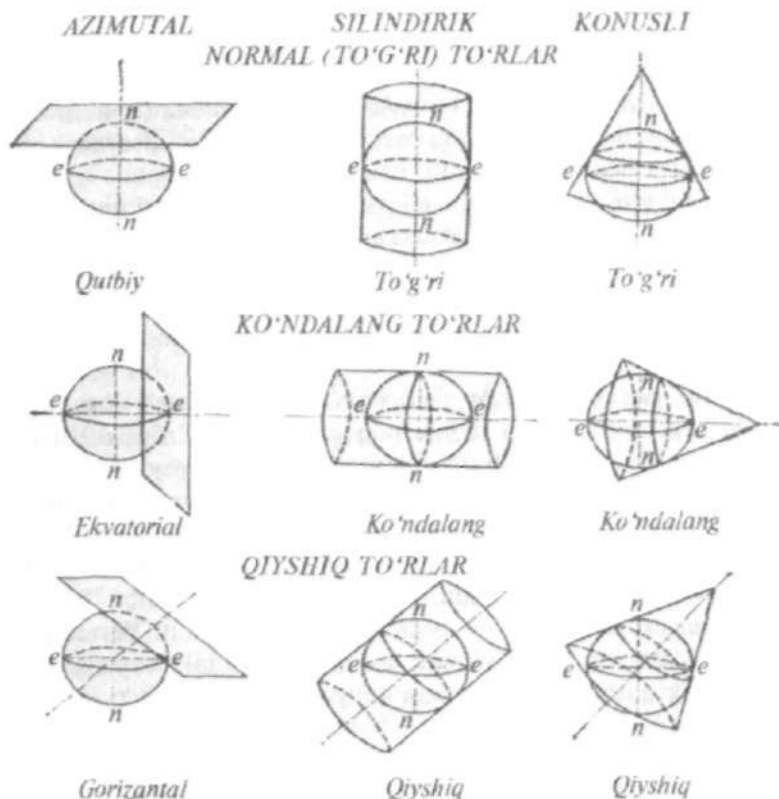
2.8-rasm. Yordamchi geometrik yuzalarni oriyentirlash.
