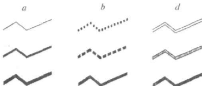
3.4-rasm. Chiziqli belgilarni bir-biridan farqlash:
