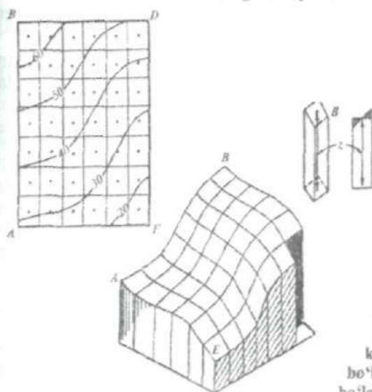
12.12- rasm. Kvadratli paletka yordamida egri chiziqlarning umumiy uzunligini aniqlash.
