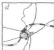
6. 1-rasm. Masshtab o'zgarishi bilan aholi punktlarini generalizatsiya qilish misolida alohida obyektlarni ularni jamlovchi belgilar bilan almashtirish:
