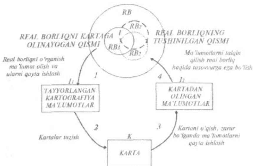
1.3-rasm. Real borliqni kartografik metod asosida bilish chizmasi:
