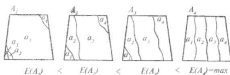
12.20-rasm. Areallar egallagan maydonlar sonini o'zgarib borishi bilan entropiyaning o'zgarishi.
