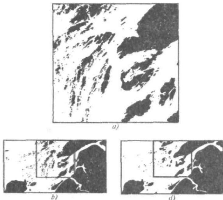
6.3-rasm. Norvegiya kartasida fiord qirg'og'ining tasviri:
