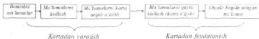
1.4-rasm. Kartografiyaning kommunikativ konsepsiyasi chizmasi.
