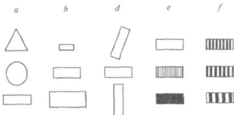
3.3-rasm. Belgilarni bir-biridan farqlash:
