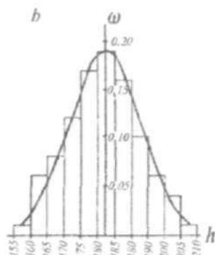
12.17-rasm. Joyning topografik kartasi va u asosida tuzilgan gistogramma. Ko'rinib turibdiki, asosiy takrorlanadigan balandliklar 180-185 m ga teng.
